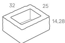
Säulenstein 25
