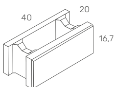
Normalstein 20
