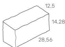
Endstein
